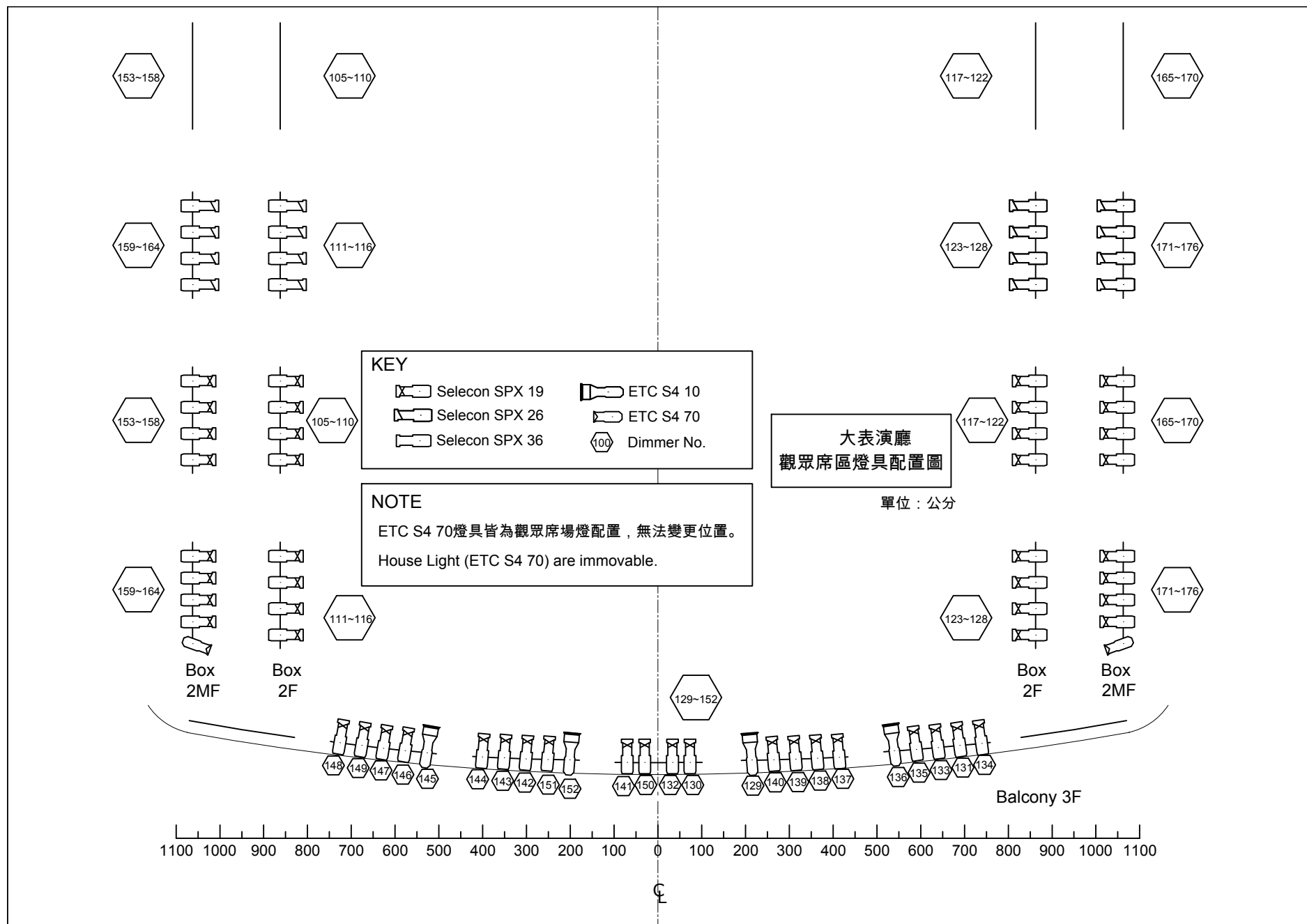
圖（十）大表演廳外區一包廂_燈具配置圖（單位：公分） Figure(10) Main Theatre - Box and Balcony__Light Plot (Unit: cm)
