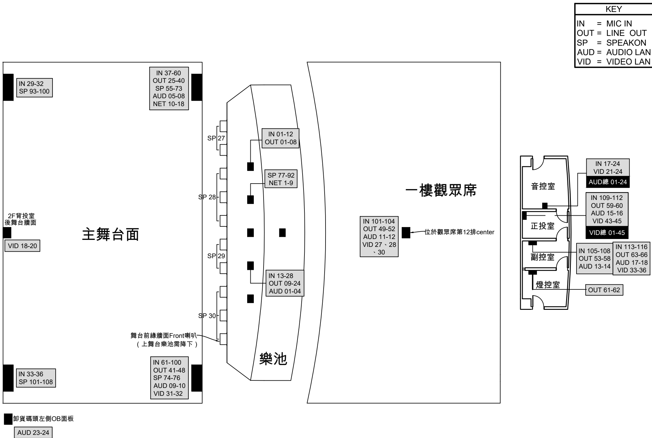
圖 (二十一) 大表演廳__ 1F音響及網絡訊號迴路圖 Figure(21) Main Theatre__ 1F Sound and Net Signal Chart
