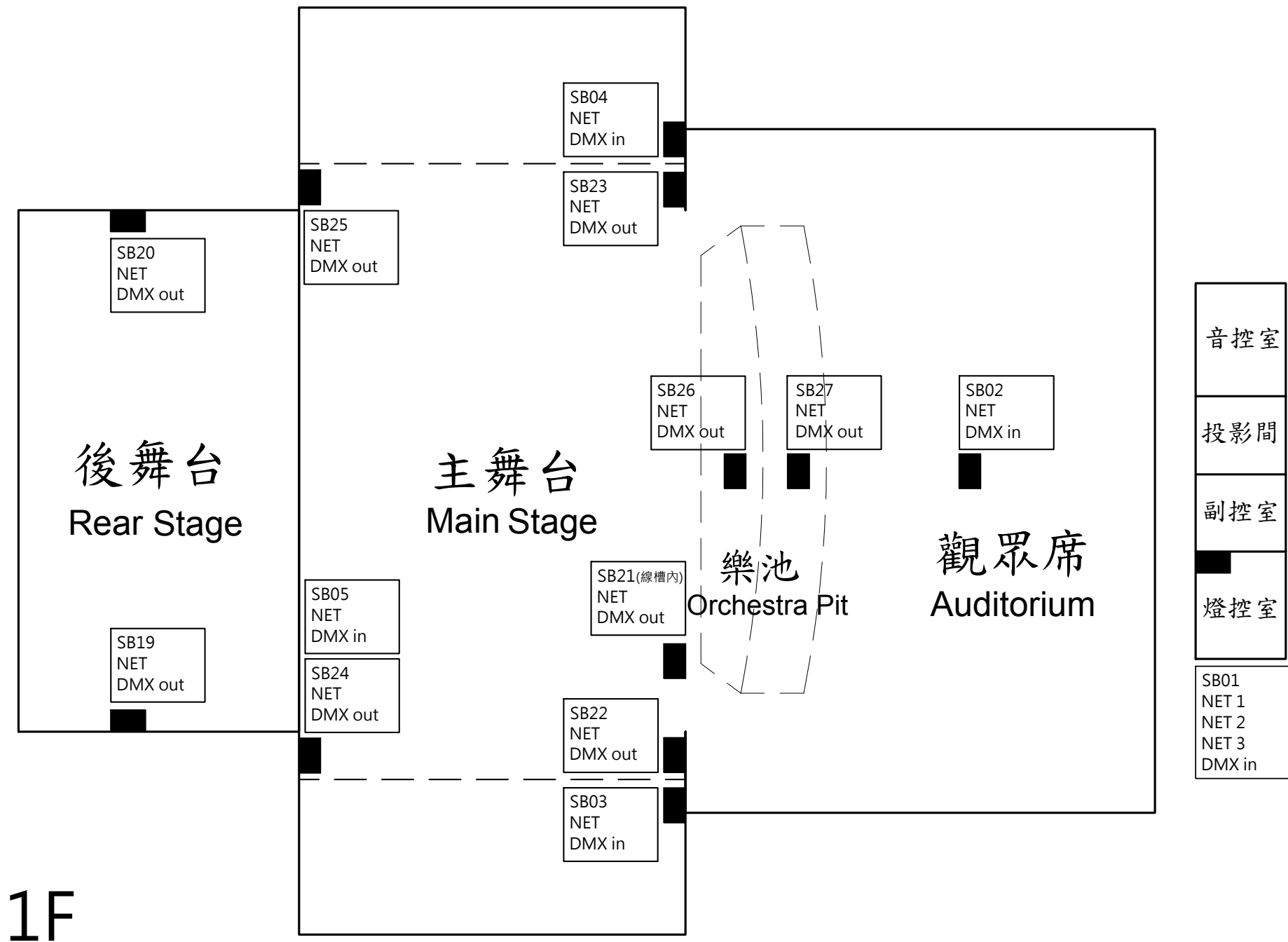
圖 (十五) 大表演廳__1F 燈光訊號盒位置圖 Figure(15) Main Theatre__1F Lighting Signal Chart
