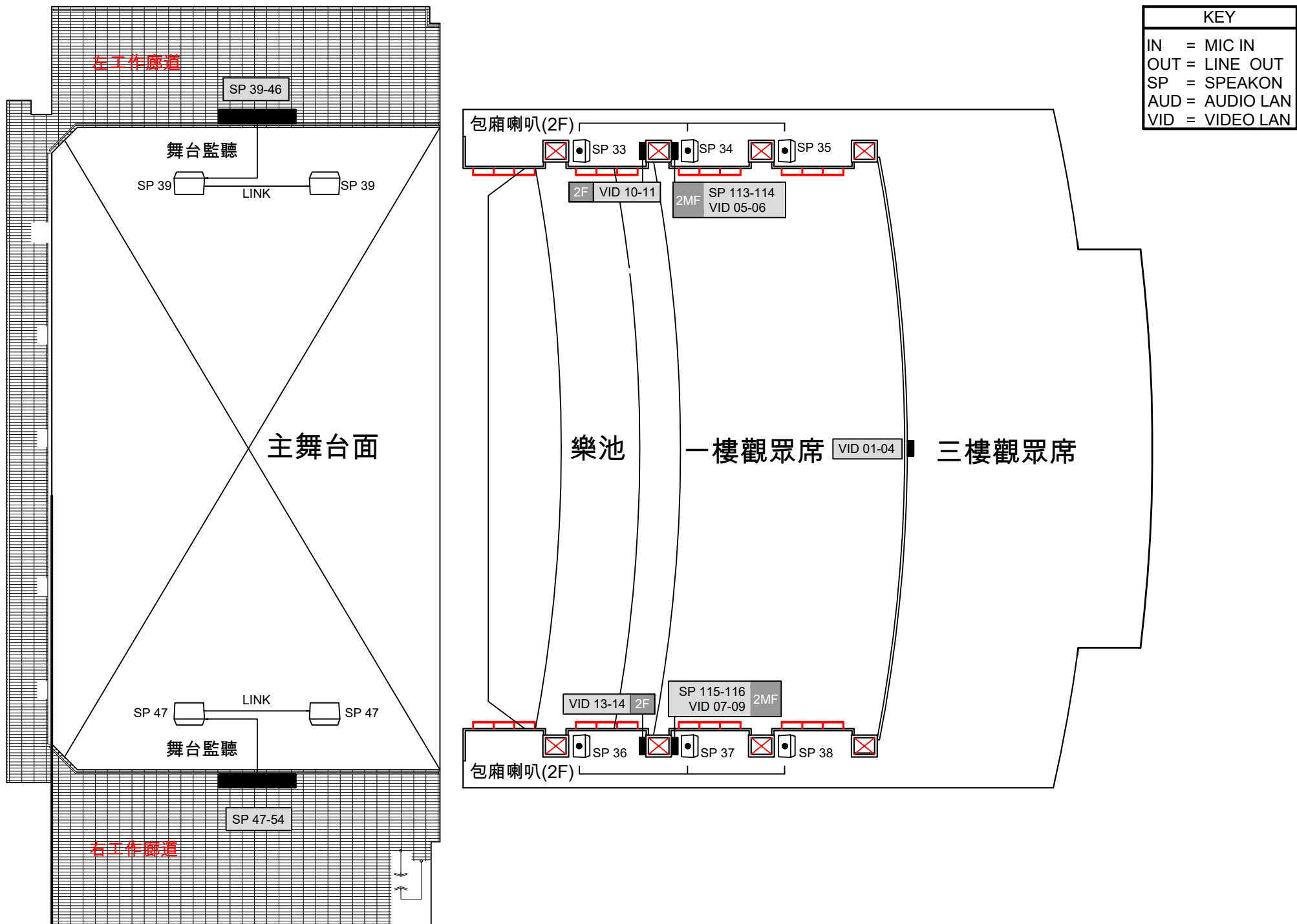
圖(二十二) 大表演廳__2F、3F音響及網路訊號迴路圖 Figure(22) Main Theatre__2F、3F Audio and Net Signal Chartz
