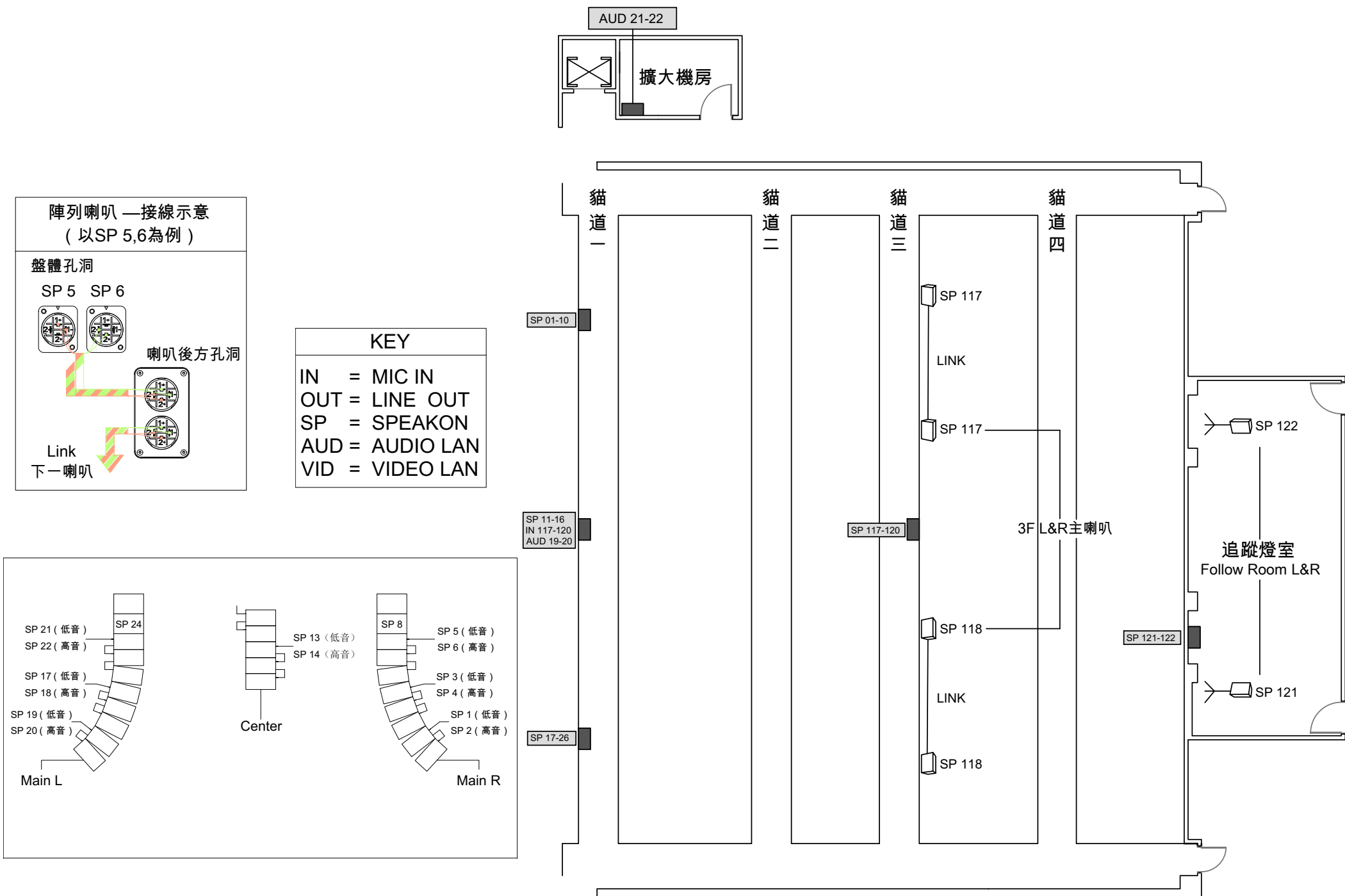
圖 (二十三) 大表演廳__ 4F音響及網絡訊號迴路圖 Figure(23) Main Theatre__ 4F Audio and Net Signal Chart
